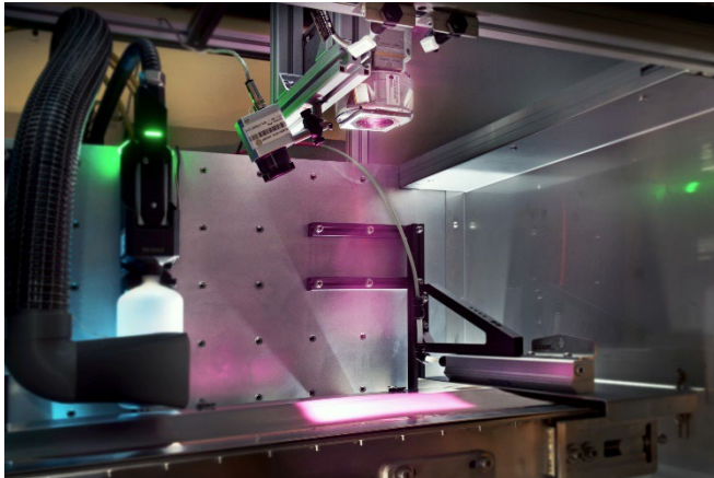
Bild 1: Die Lasertrocknung im Rolle-zu-Rolle-Verfahren macht die Serienproduktion von Lithium-Ionen-Batterien deutlich nachhaltiger und wirtschaftlicher. Dafür wurde im IDEEL Forschungsprojekt ein Hochleistungsdiodelaser mit Zoomoptik in eine Folienbeschichtungsanlage integriert. © Fraunhofer ILT, Aachen.
